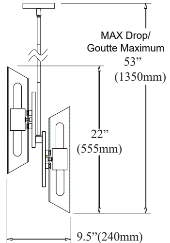
Side view Vue de côté
