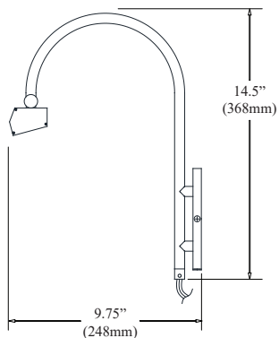
Side view Vue de côté
