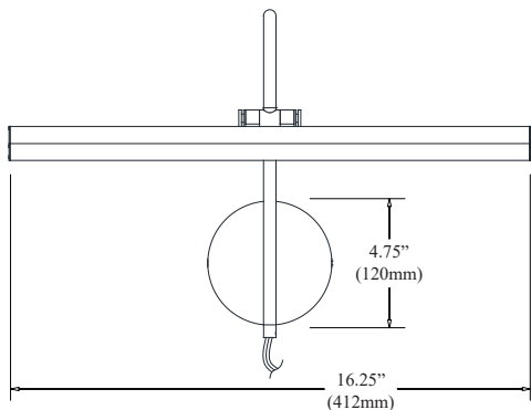
Front view Vue de face
